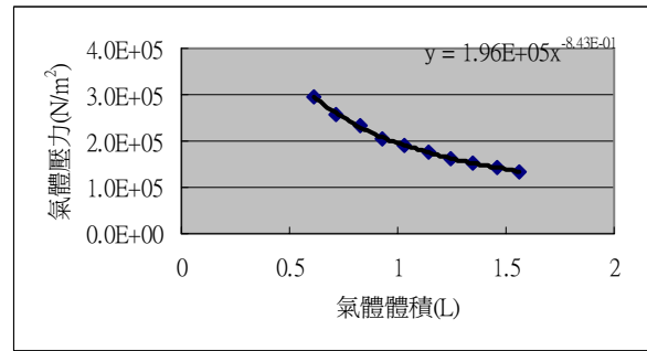
圖 7-4 2L 鹽水氣體體積與容器氣壓關係
