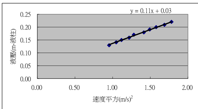
圖 6-2 2L 開放式容器鹽水噴射速度平方與液壓關係
