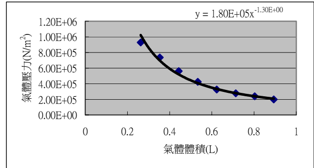
圖 7-6 1.320L 水氣體體積與容器氣壓關係
