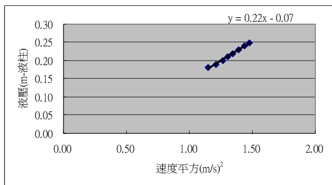
圖 6-3 1.320L 開放式容器水噴射速度平方與液壓關係
