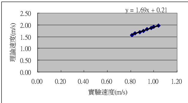
圖 7-7 0.683L 水--實驗速度與理論速度關係
