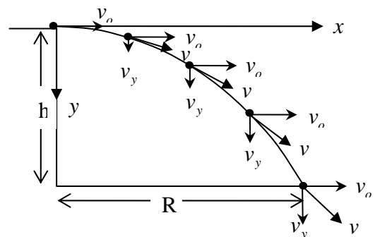
圖 5-1 水平拋射運動的軌跡
