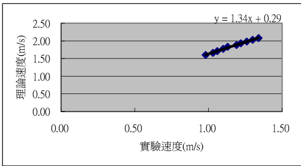
圖 7-3 2L 鹽水實驗速度與理論速度關係
