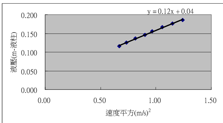
圖 6-5 2L 開放式容器水噴射速度與液壓關係
