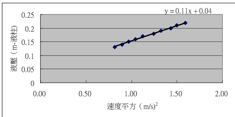
圖 6-1 2L 開放式容器水噴射速度平方與液壓關係
