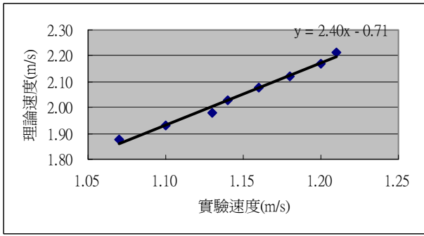
圖 7-5 1.320L 水實驗速度與理論速度關係
