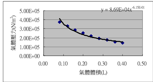
圖 7-8 0.683L 水--氣體體積與容器氣壓關係
