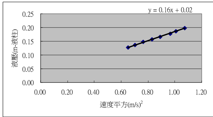
圖 6-4 683mL 開放式容器水噴射速度平方與液壓關係
